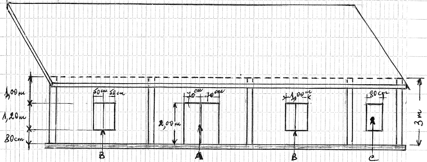
VUE DE DROITE
